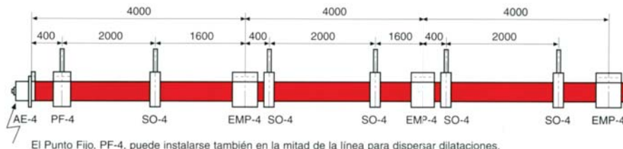
LÍNEA EN INTERIOR CON ALIMENTACION EXTREMA (Soportes cada 2 metros)
