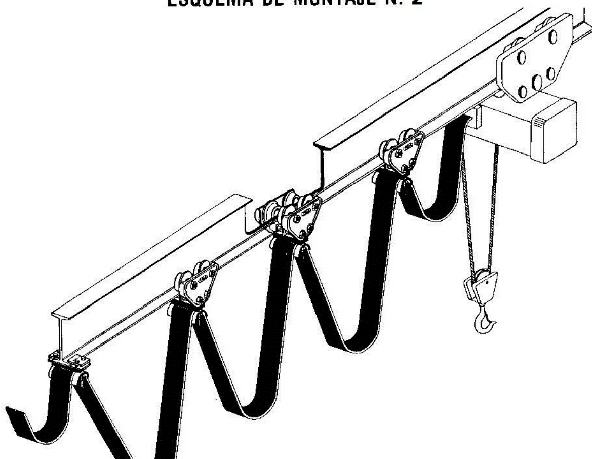
ESQUEMA DE MONTAJE N° 2
