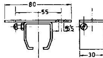
Soporte - Ref. 2.401-4-A (Con prisionero)
