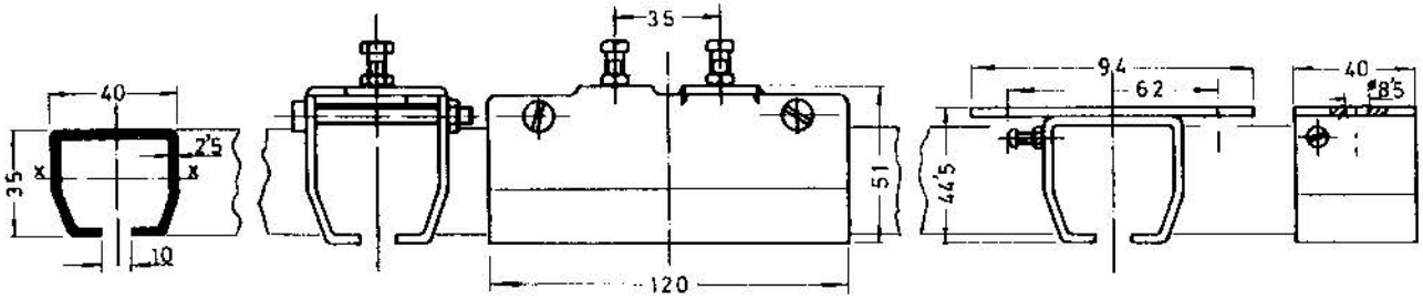
Perfil - Ref. 2.500-150-1
